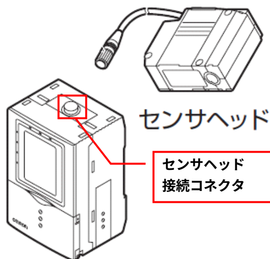
(センサコントローラ上面)
