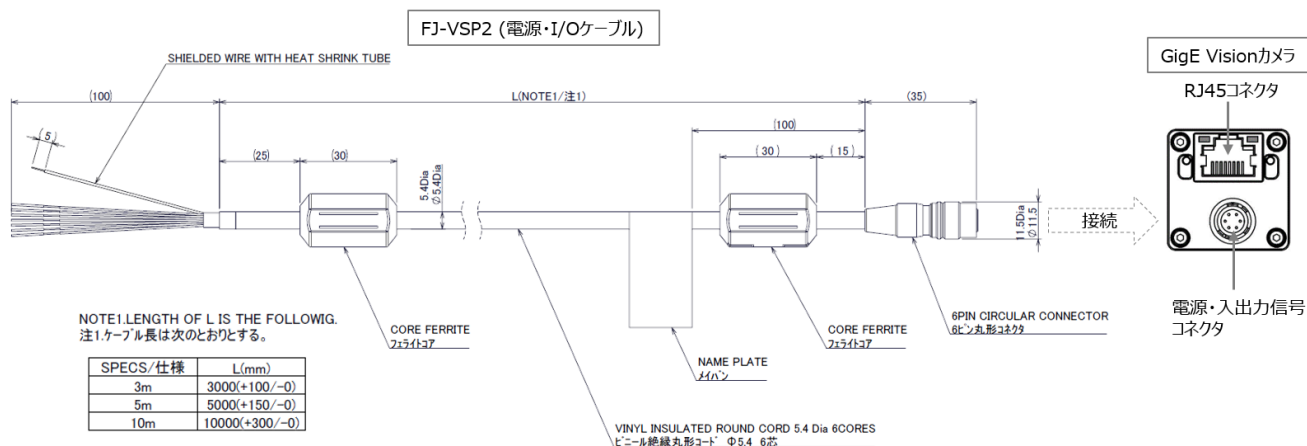
接続図
