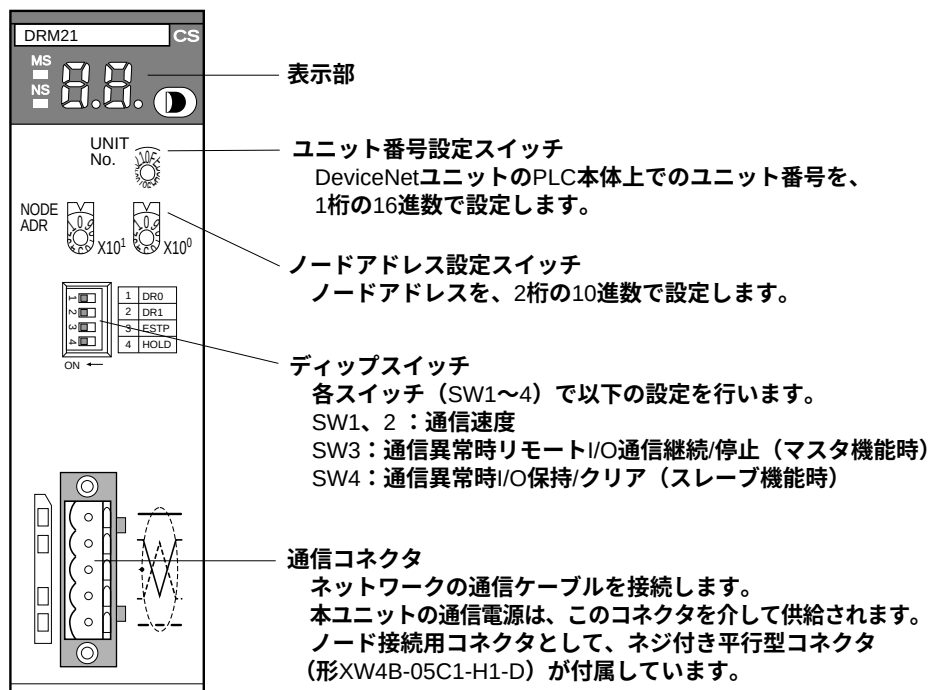
形 CS1W-DRM21(-V1)
