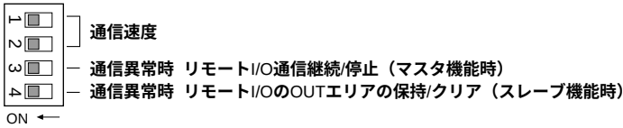
形CJ1W-DRM21
