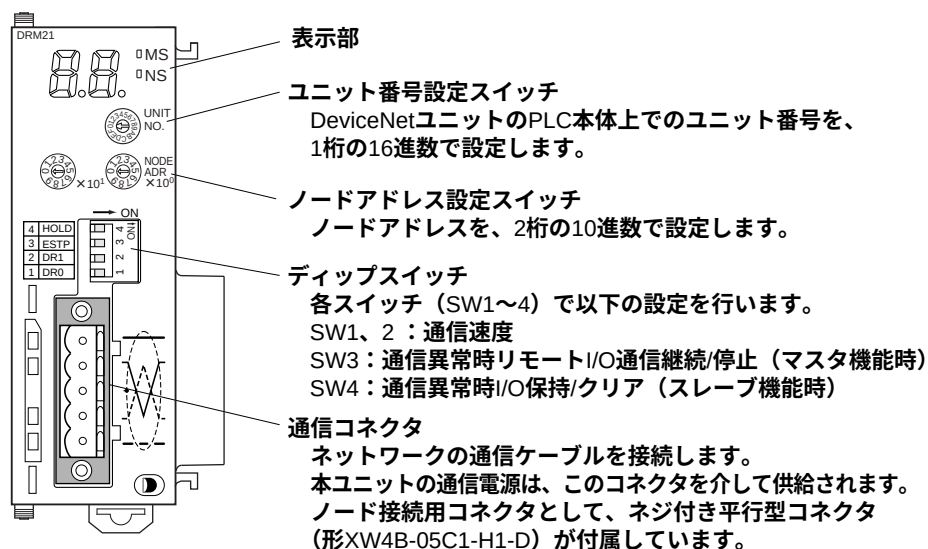
形 CJ1W-DRM21
