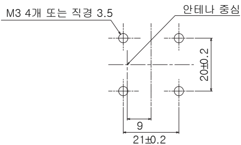
장착 치수
