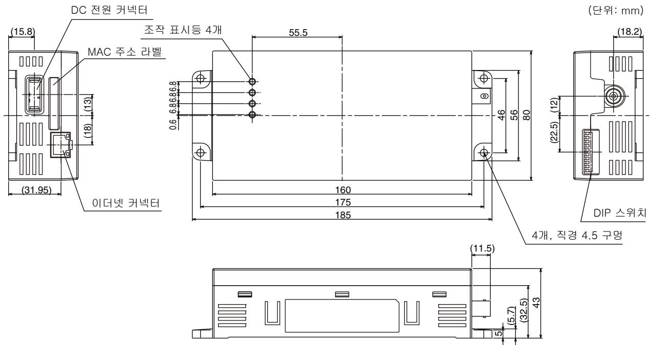
장착 치수
