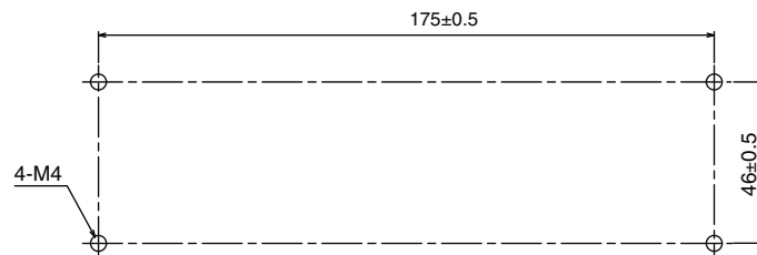
장착 치수
